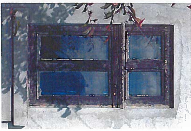
Balra: egyszerű homlokzati felületen díszes, 4 osztott tokos, téglapárkányos ablak. Középen: kifelé és befelé nyíló ablakszármnyakkal rendelkező nyílászáró. Jobbra: vakolt párkányos 4 osztott tokú ablak.
